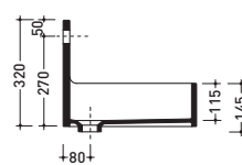
sezione longitudinale / section
