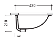
sezione longitudinale / section
