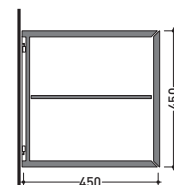
sezione longitudinale / section
