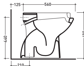
sezione longitudinale / section
