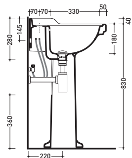
sezione longitudinale / section
