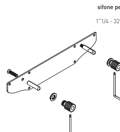
SISTEMA DI FISSAGGIO / FIXING SYSTEM IN DOTAZIONE / INCLUDED IN THE BOX
