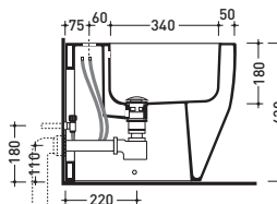
sezione longitudinale / section
