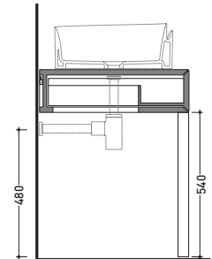
sezione longitudinale / section
