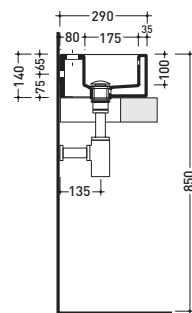
sezione longitudinale / section
