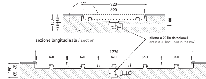
sezione trasversale / section
