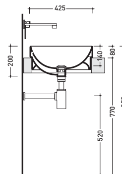
sezione longitudinale / section
