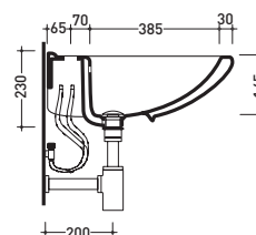
sezione longitudinale / section
