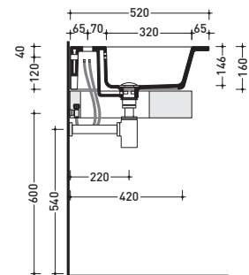
sezione longitudinale / section
