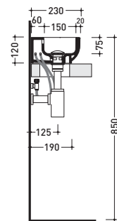
sezione longitudinale / section
