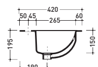
sezione longitudinale / section
