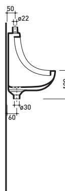
sezione longitudinale / section
