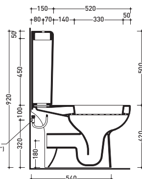
sezione longitudinale / section
