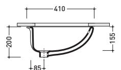
sezione longitudinale / section
