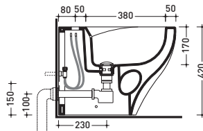
sezione longitudinale / section
