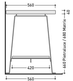
sezione longitudinale / section
