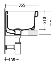
sezione longitudinale / section
