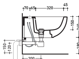
sezione longitudinale / section
