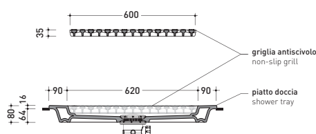
sezione longitudinale / section
