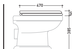
sezione longitudinale / section
