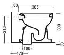
sezione longitudinale / section
