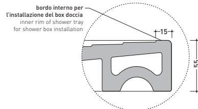
dettaglio del bordo / shower tray rim detail
