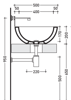
sezione longitudinale / section
