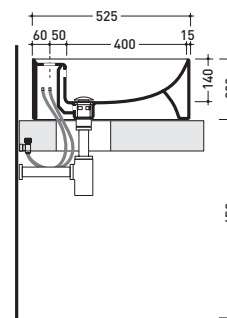
sezione longitudinale / section
