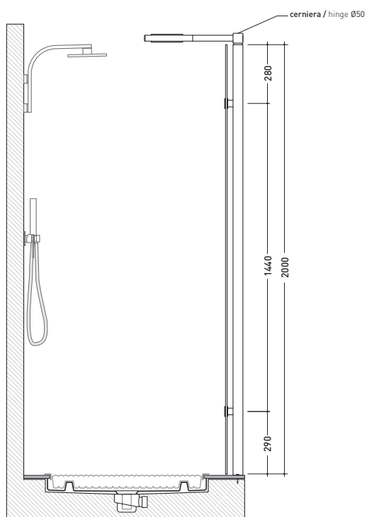
sezione longitudinale / section
