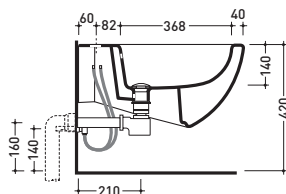
sezione longitudinale / section
