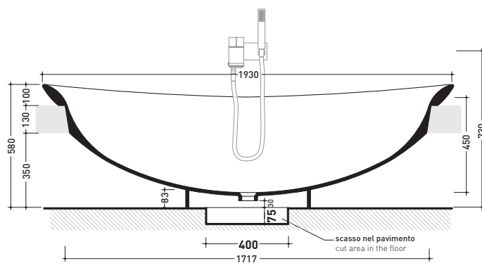
sezione longitudinale / section
