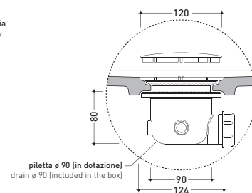
dettaglio piletta / drain detail
