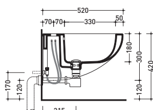
sezione longitudinale / section
