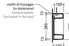
sezione longitudinale / section
