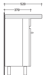
sezione longitudinale / section
