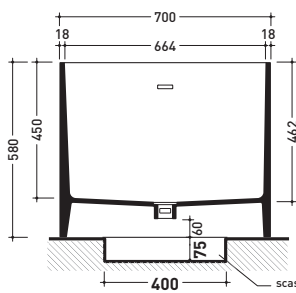
sezione laterale / section
