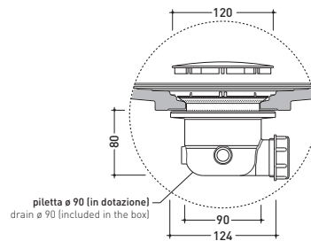
dettaglio piletta / drain detail
