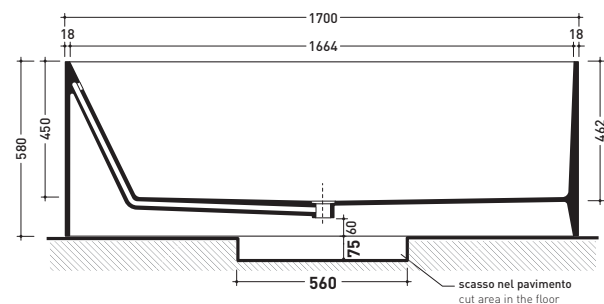
sezione longitudinale / section
