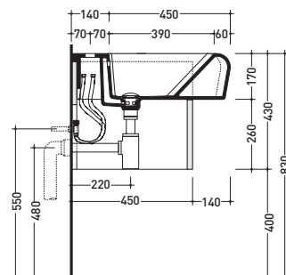
sezione longitudinale / section
