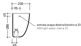
sezione longitudinale / section
