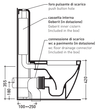
sezione longitudinale / section
