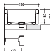
sezione longitudinale / section
