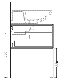
sezione longitudinale / section
