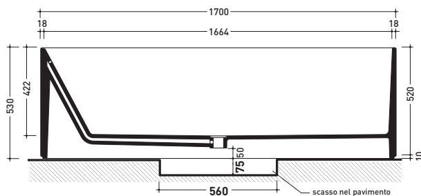
sezione longitudinale / section
