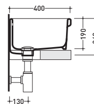
sezione longitudinale / section
