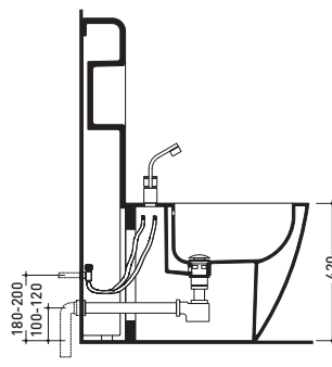
sezione longitudinale / section
