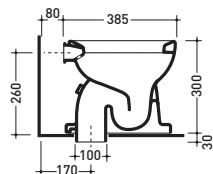
sezione longitudinale / section
