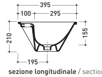
sezione longitudinale / section
