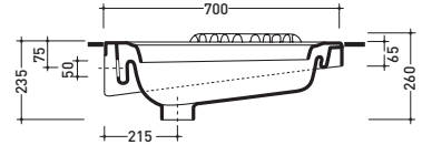
sezione longitudinale / section
