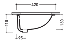
sezione longitudinale / section
