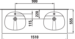
1467.8 Doppelwaschtisch unterbaufähig Double countertop washbasin Lavabo double à poser sur meuble Lavabo consolle, doppio bacino
