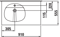
1467.1 Waschtisch asymmetrisch unterbaufähig, Ablage rechts Asymmetrical countertop washbasin, basin left Lavabo asymétrique à poser sur meuble, tablette à droite Lavabo consolle asimmetrico, bacino a sinistra
