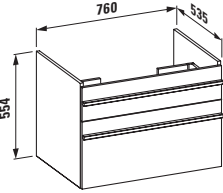
2432.1 Waschtischunterbau asymmetrisch links, passend zu Waschtisch 1467.1, 1 Türe, 1 Ablage, 2 Schubladen
