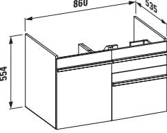
2432.2 Waschtischunterbau asymmetrisch rechts, passend zu Waschtisch 1467.2, 1 Türe, 1 Ablage, 2 Schubladen
