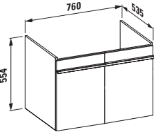
2430.4 Waschtischunterbau passend zu Waschtisch 1467.0, 2 Schubladen
