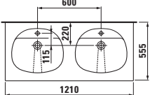
1467.7 Doppelwaschtisch unterbaufähig Double countertop washbasin Lavabo double à poser sur meuble Lavabo consolle, doppio bacino
