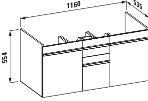
Base sottolavabo per lavabo 1467.7, 2 ante, 2 ripiani, 2 cassetti
