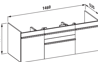
Base sottolavabo per lavabo 1467.8, 2 ante, 2 ripiani, 2 cassetti
